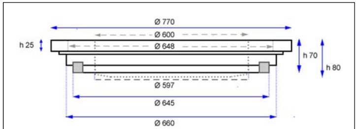
Skizze Swiss-Edition DN 600 35kN mit CH-Modulrahmen – Abmessungen ca. Angaben.
