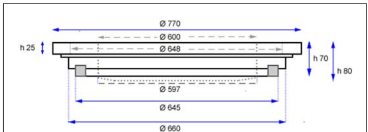
Skizze Swiss-Edition DN 600 35kN mit CH-Modulrahmen – Abmessungen ca. Angaben.
